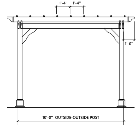
RIGHT ELEVATION
